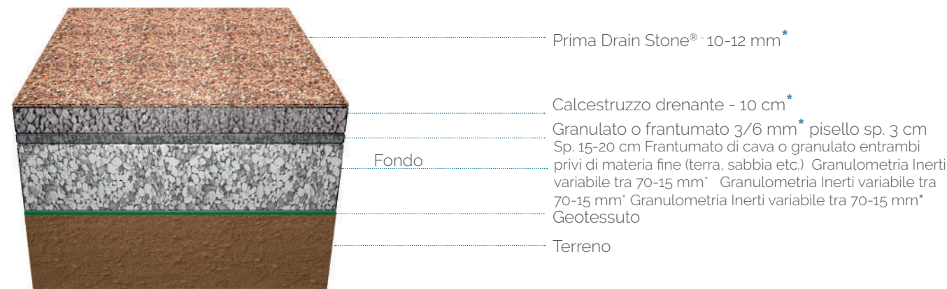
Prima Drain Stone® su fondo calcestruzzo permeabile - Pedonale e ciclabile * Valori nominali
