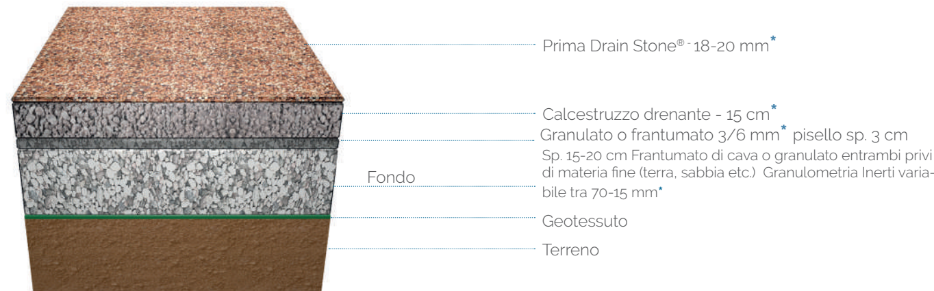
Prima Drain Stone® su fondo calcestruzzo permeabile - versione carrabile (≤ 3,5 ton) * Valori nominali
